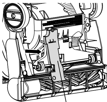
Cubierta de la correa
